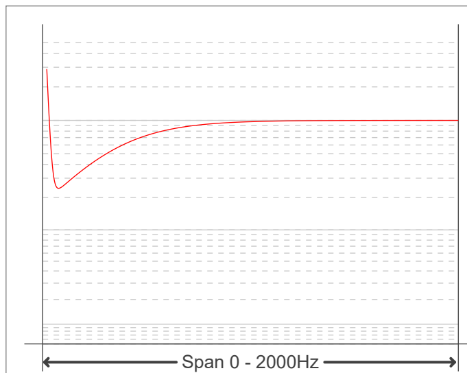
Flickr FFT (průběh flickru v závislosti na frekvenci)
