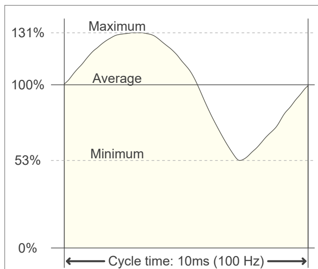
Průběh flikru (průběh jedné periody flikru v čase)
