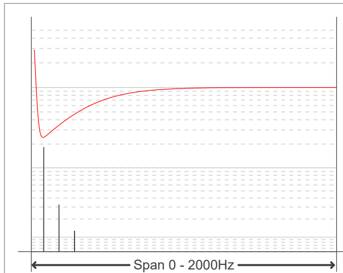
Flikr FFT (průběh flikru v závislosti na frekvenci)
